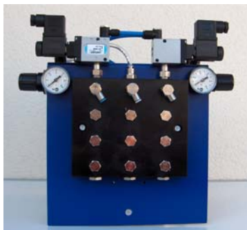
Standard-Sprühgerät mit Angebauter Ventil- und Verteilerplatte
